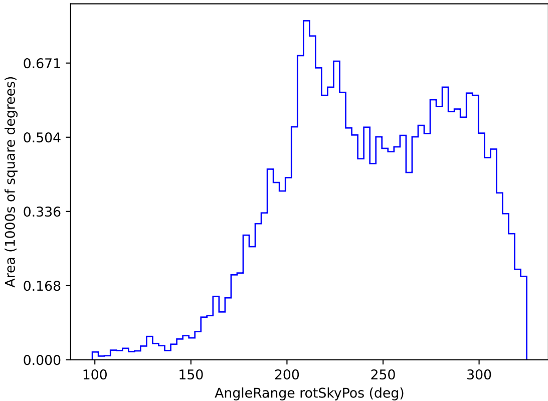
extra_ss_neo4_v3.4_10yrs All sky u band: AngleRange rotSkyPos
