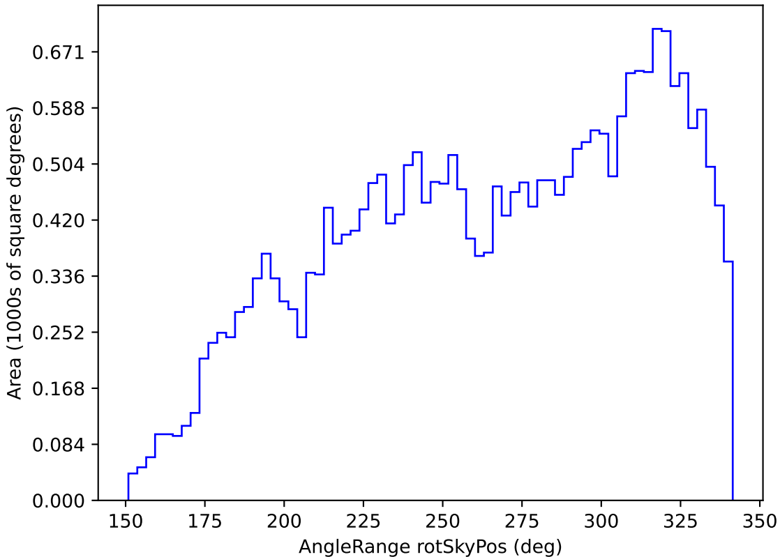
extra_ss_neo4_v3.4_10yrs All sky i band: AngleRange rotSkyPos
