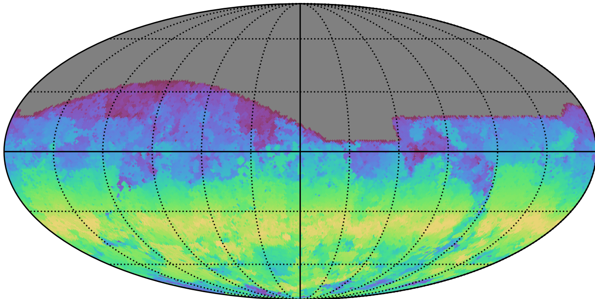
extra_ss_neo4_v3.4_10yrs All sky g band: AngleRange rotSkyPos
