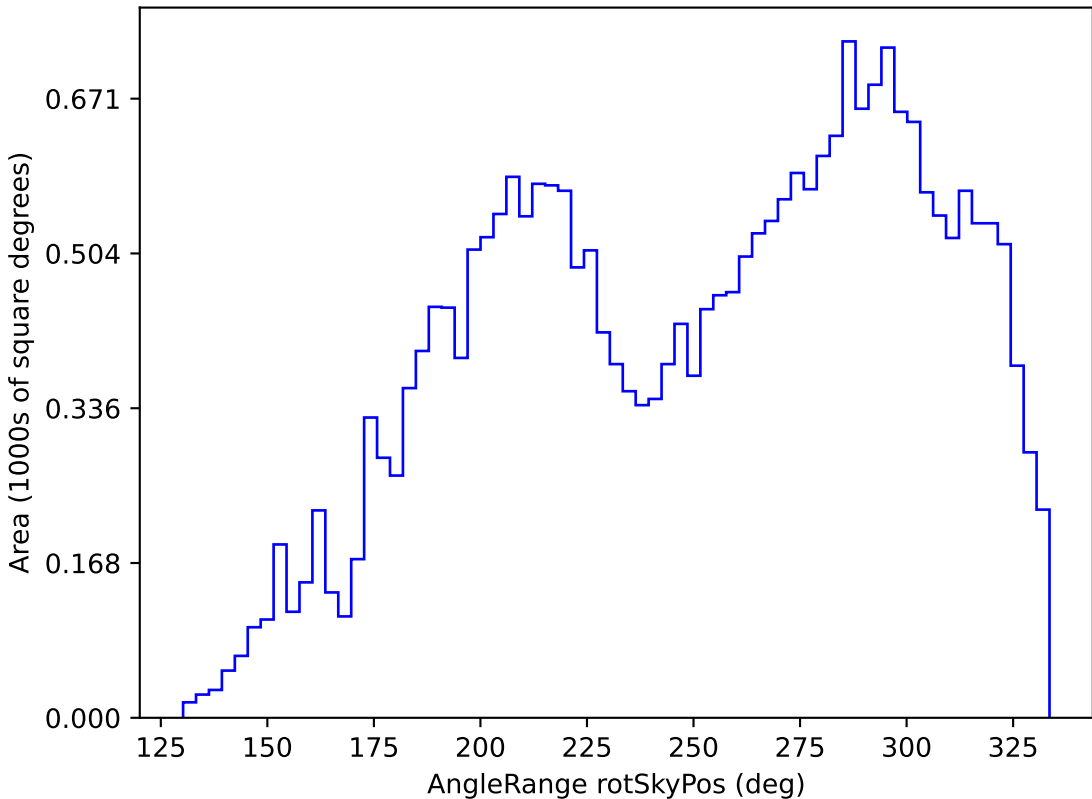
extra_ss_neo4_v3.4_10yrs All sky g band: AngleRange rotSkyPos
