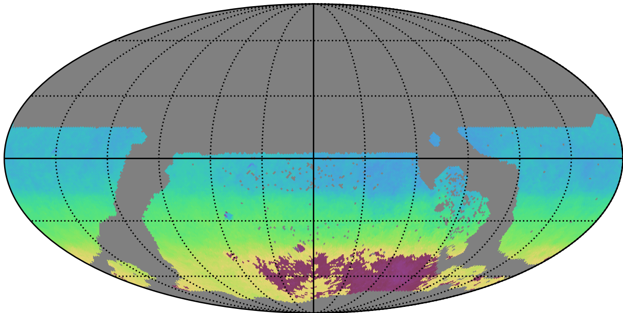
extra_ss_neo4_v3.4_10yrs WFD y band: AngleMean rotSkyPos
