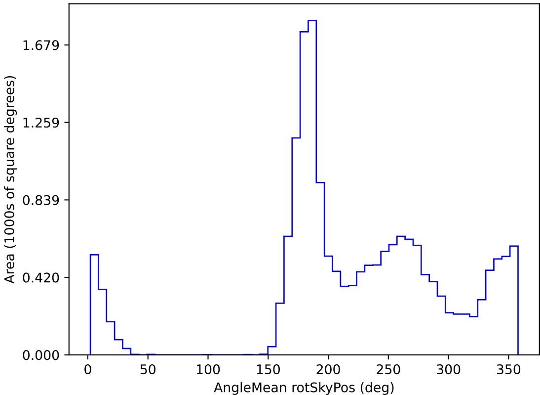
extra_ss_neo4_v3.4_10yrs WFD y band: AngleMean rotSkyPos
