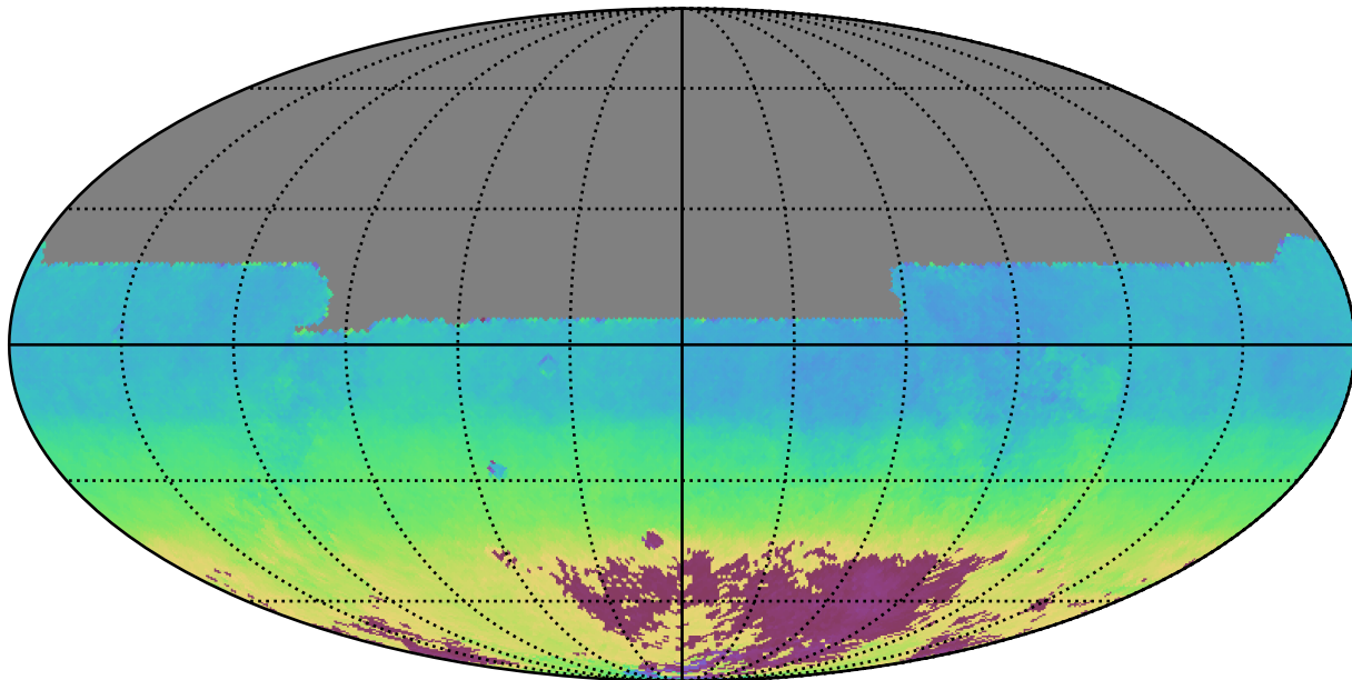
extra_ss_neo4_v3.4_10yrs All sky y band: AngleMean rotSkyPos
