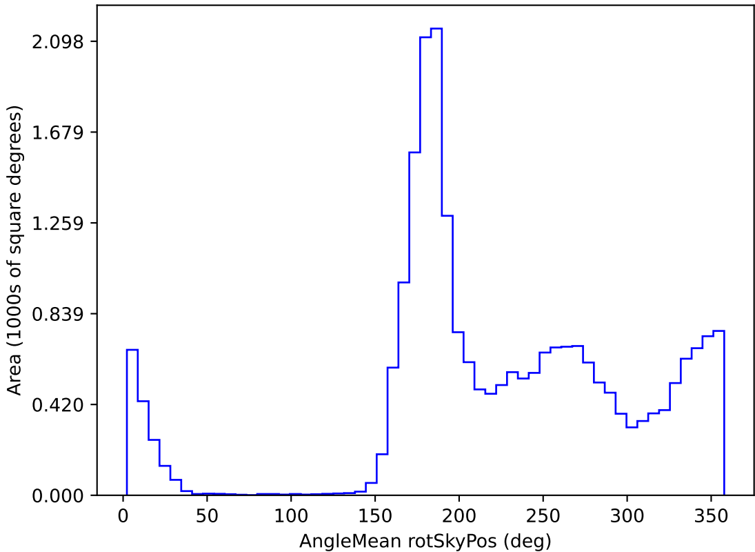
extra_ss_neo4_v3.4_10yrs All sky y band: AngleMean rotSkyPos
