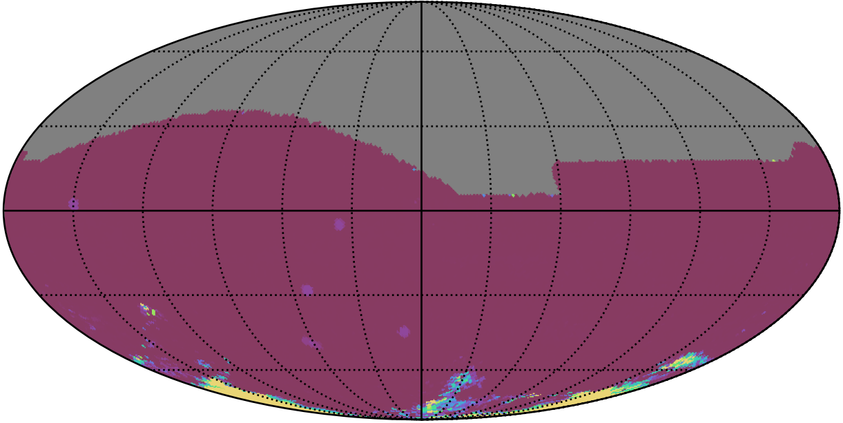
extra_ss_neo4_v3.4_10yrs All sky iz bands: 75th Percentile Intranight Timespan
