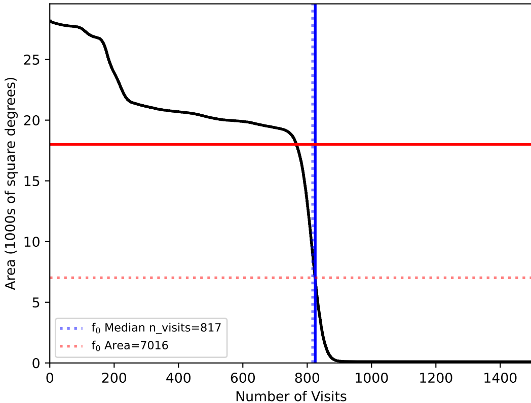
extra_ss_neo4_v3.4_10yrs : f0
