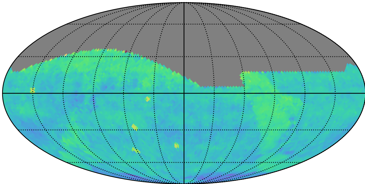
extra_ss_neo4_v3.4_10yrs (g or r or i): PairFraction
