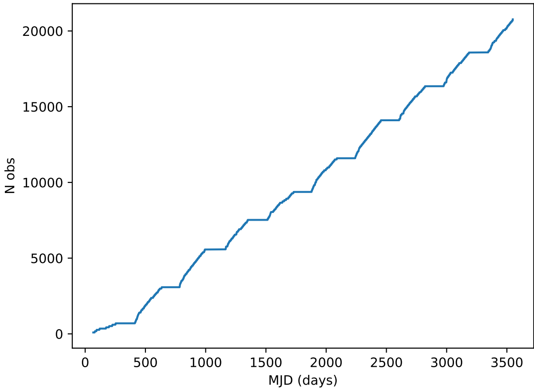
extra_ss_neo4_v3.4_10yrs note like DD:ELAISS1%: Cumulative
