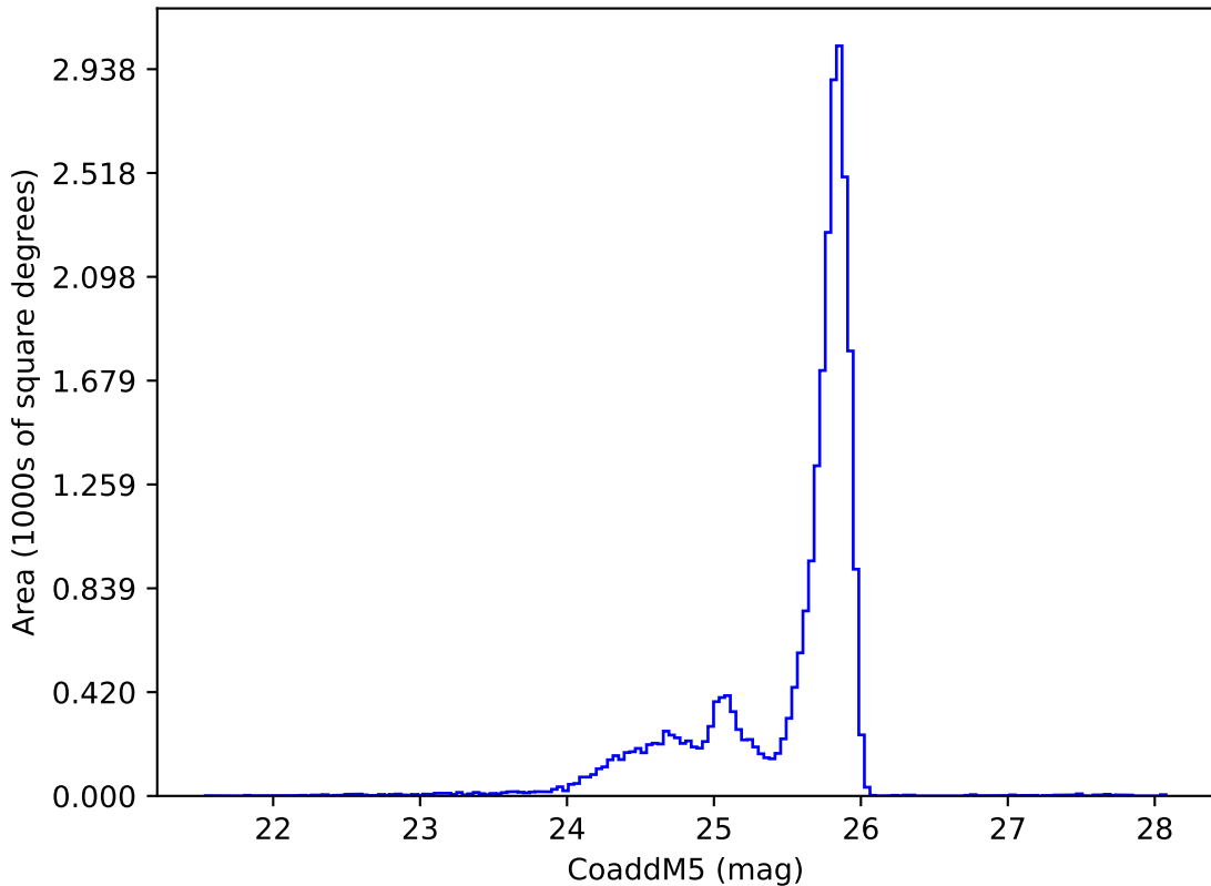
extra_ss_neo4_v3.4_10yrs z: CoaddM5
