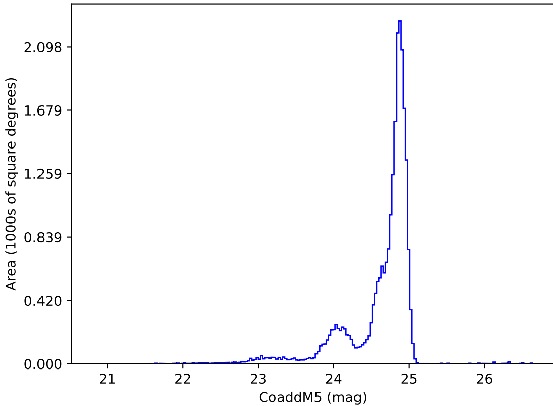
extra_ss_neo4_v3.4_10yrs y: CoaddM5
