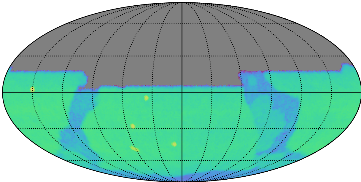
extra_ss_neo4_v3.4_10yrs u: CoaddM5
