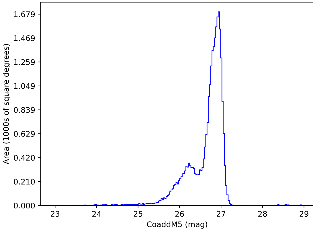
extra_ss_neo4_v3.4_10yrs g: CoaddM5
