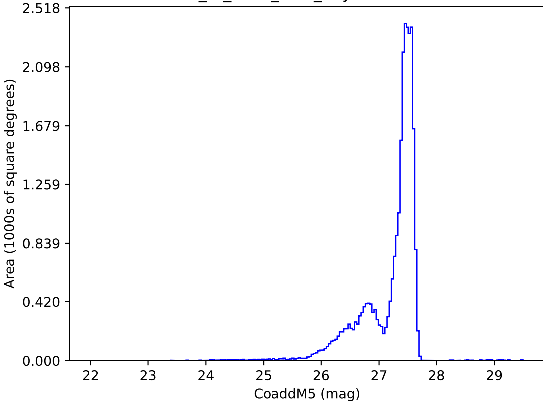
extra_ss_neo4_v3.4_10yrs : CoaddM5
