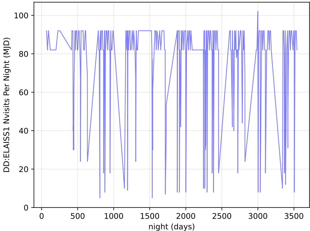
extra_ss_neo4_v3.4_10yrs all bands: DD:ELAISS1 Nvisits Per Night
