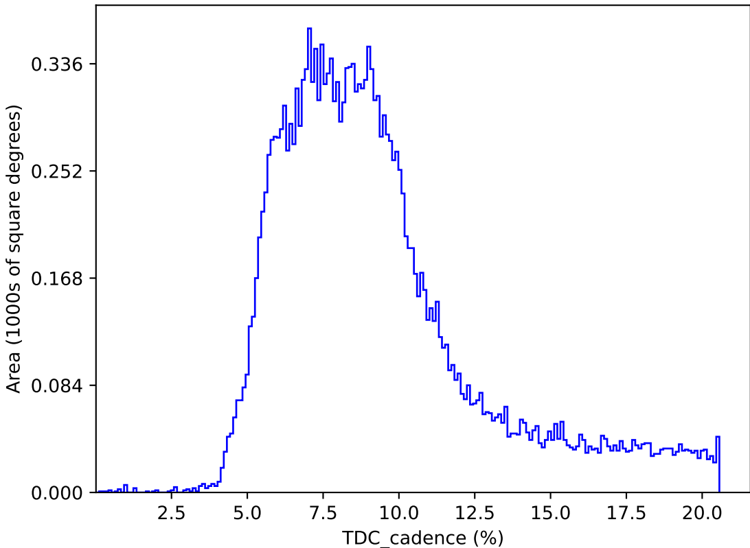
extra_ss_neo3_v3.4_10yrs : TDC_cadence
