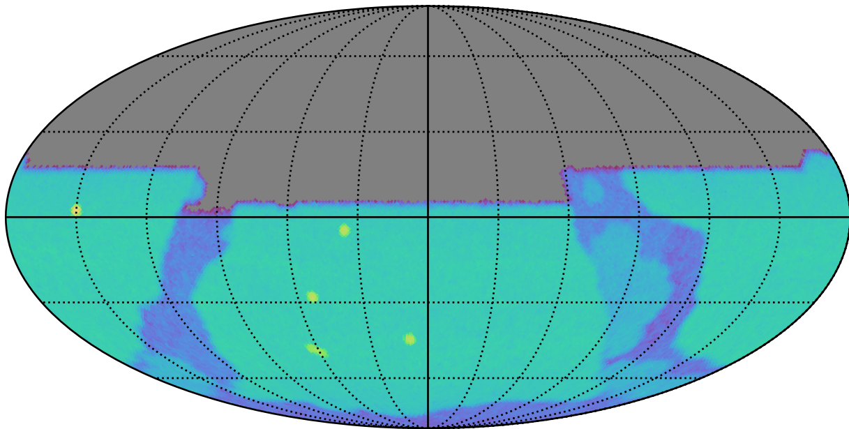
extra_ss_neo3_v3.4_10yrs u: SurfaceBrightLimit
