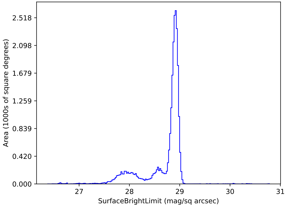
extra_ss_neo3_v3.4_10yrs u: SurfaceBrightLimit
