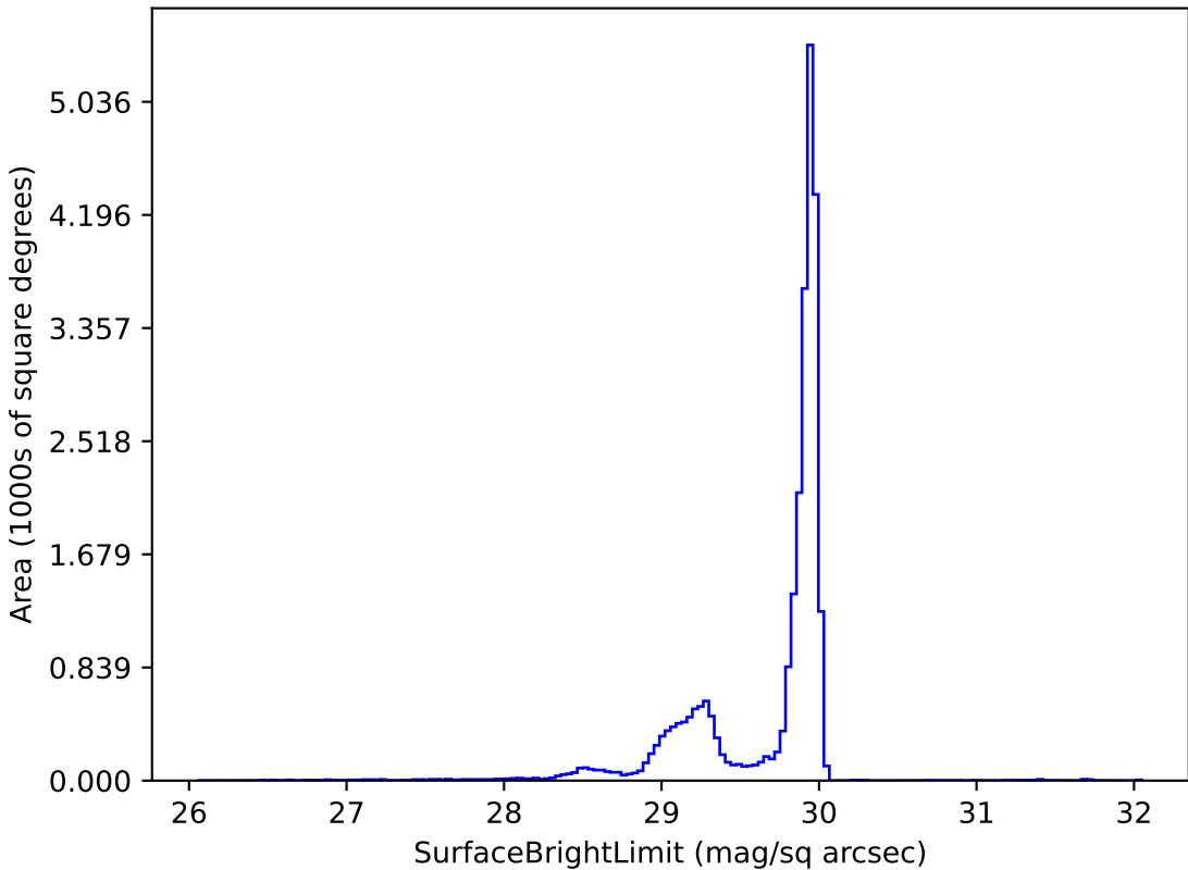
extra_ss_neo3_v3.4_10yrs i: SurfaceBrightLimit
