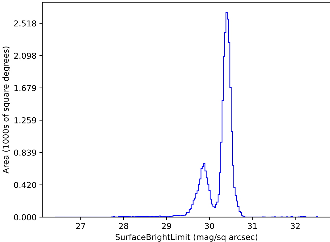
extra_ss_neo3_v3.4_10yrs g: SurfaceBrightLimit
