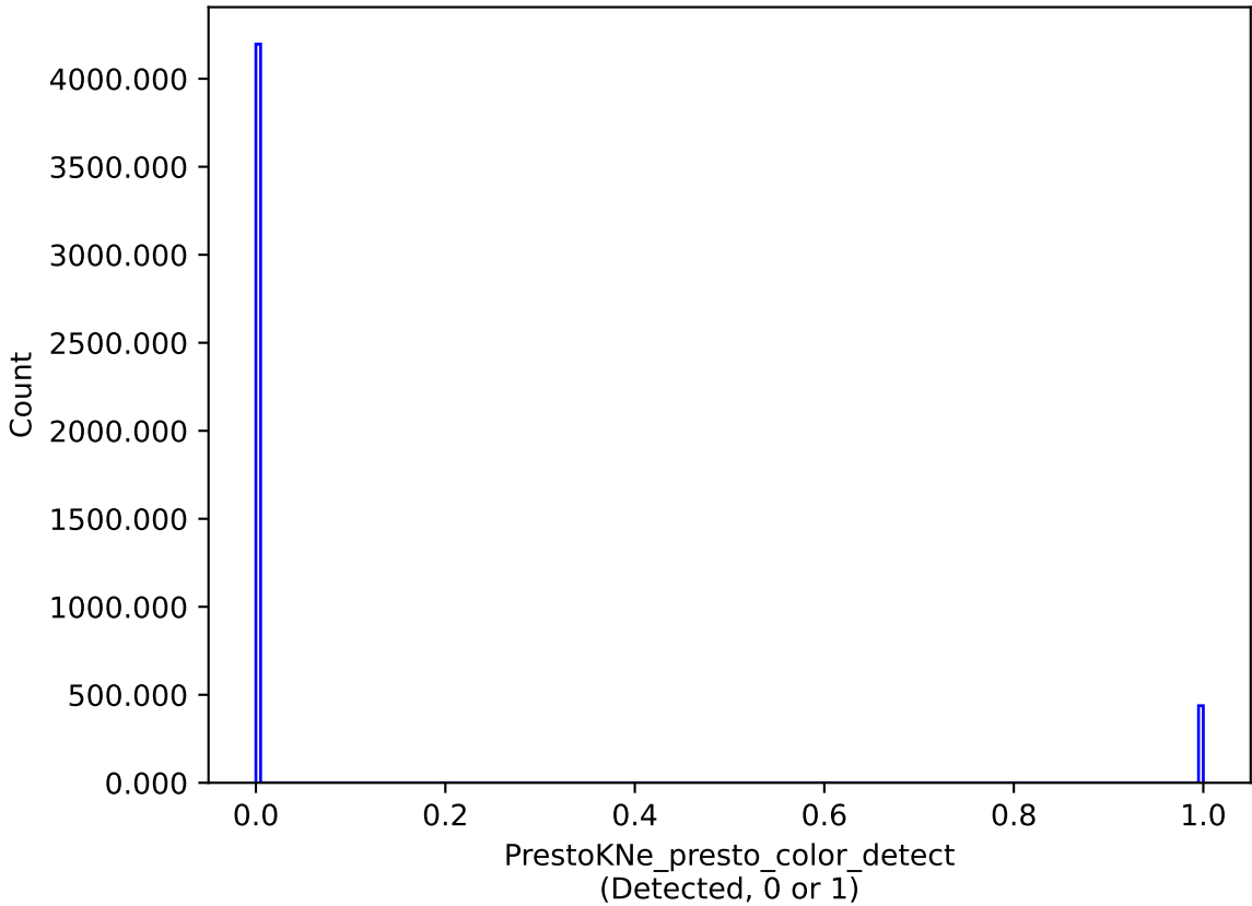
extra_ss_neo3_v3.4_10yrs : PrestoKNe_presto_color_detect
