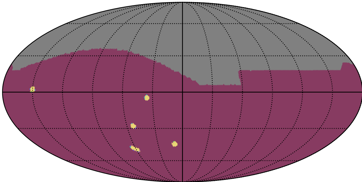
extra_ss_neo3_v3.4_10yrs : NumberOfQuickRevisits
