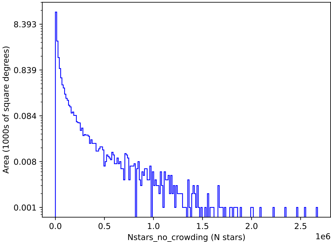
extra_ss_neo3_v3.4_10yrs u: Nstars_no_crowding
