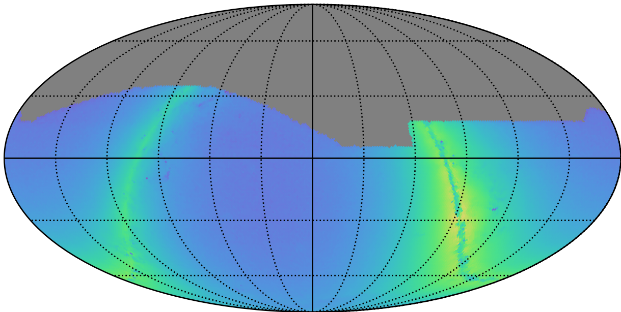
extra_ss_neo3_v3.4_10yrs r: Nstars_no_crowding
