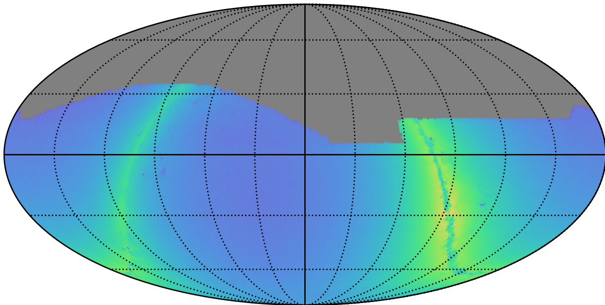
extra_ss_neo3_v3.4_10yrs i: Nstars_no_crowding
