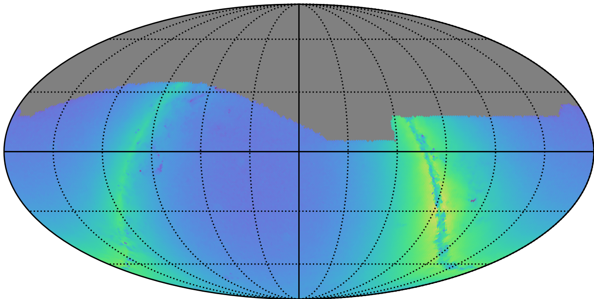
extra_ss_neo3_v3.4_10yrs g: Nstars_no_crowding
