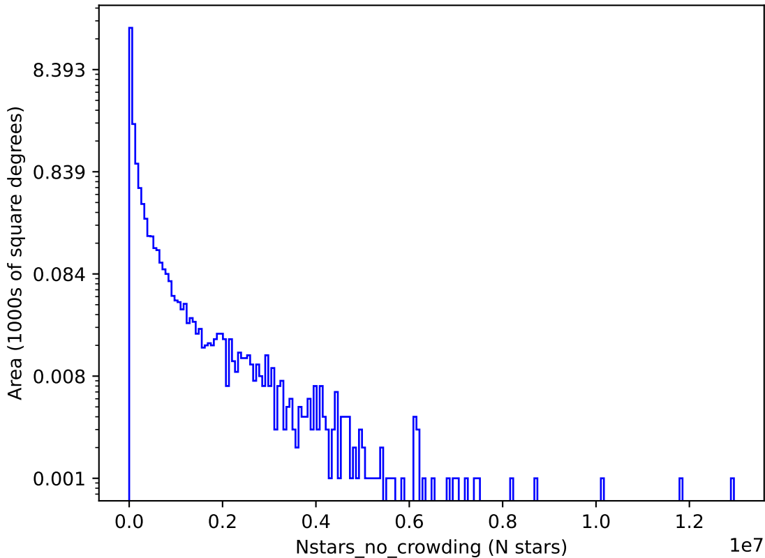
extra_ss_neo3_v3.4_10yrs g: Nstars_no_crowding
