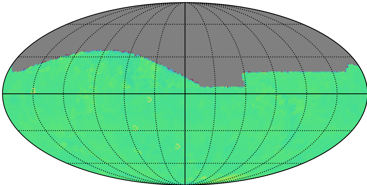
extra_ss_neo3_v3.4_10yrs z: Kuiper rotTelPos
