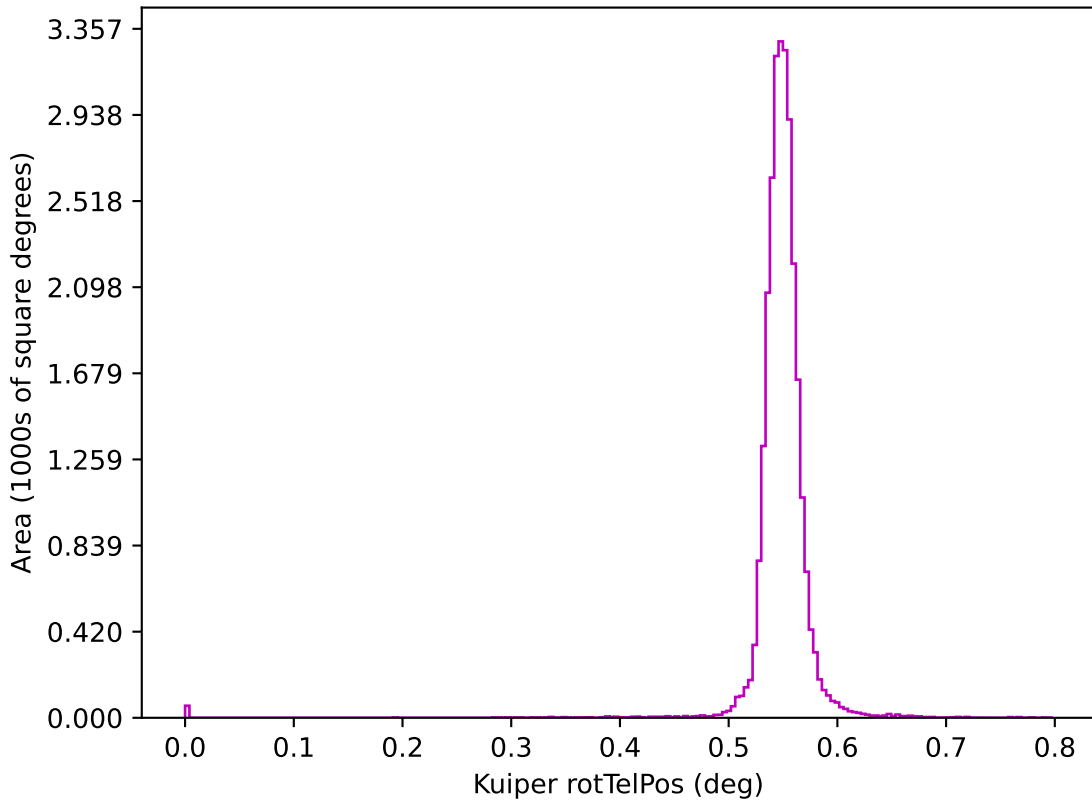
extra_ss_neo3_v3.4_10yrs z: Kuiper rotTelPos
