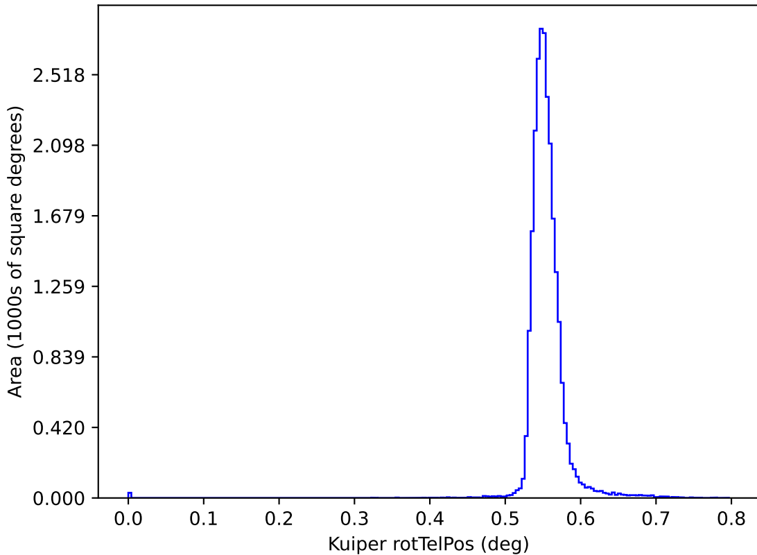
extra_ss_neo3_v3.4_10yrs y: Kuiper rotTelPos
