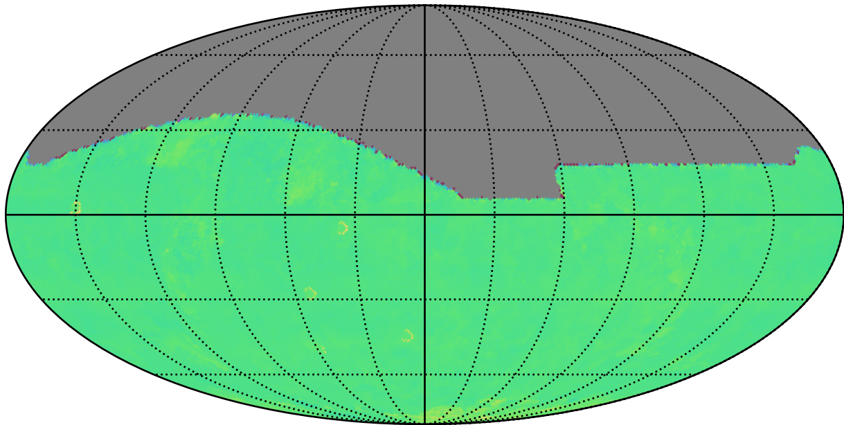
extra_ss_neo3_v3.4_10yrs r: Kuiper rotTelPos
