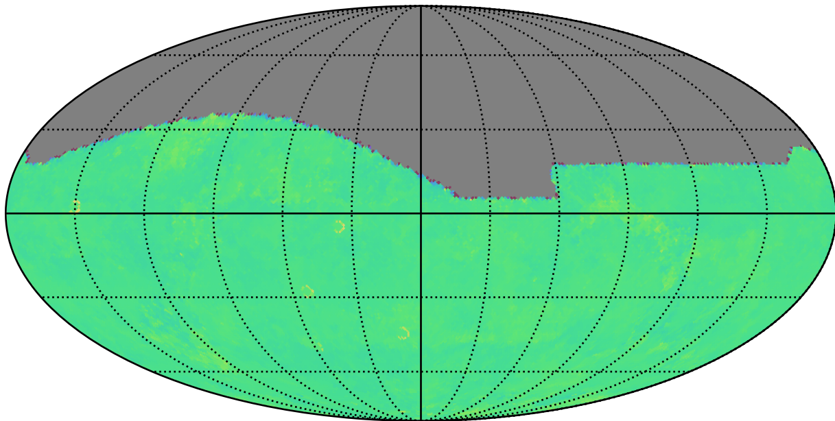
extra_ss_neo3_v3.4_10yrs g: Kuiper rotTelPos
