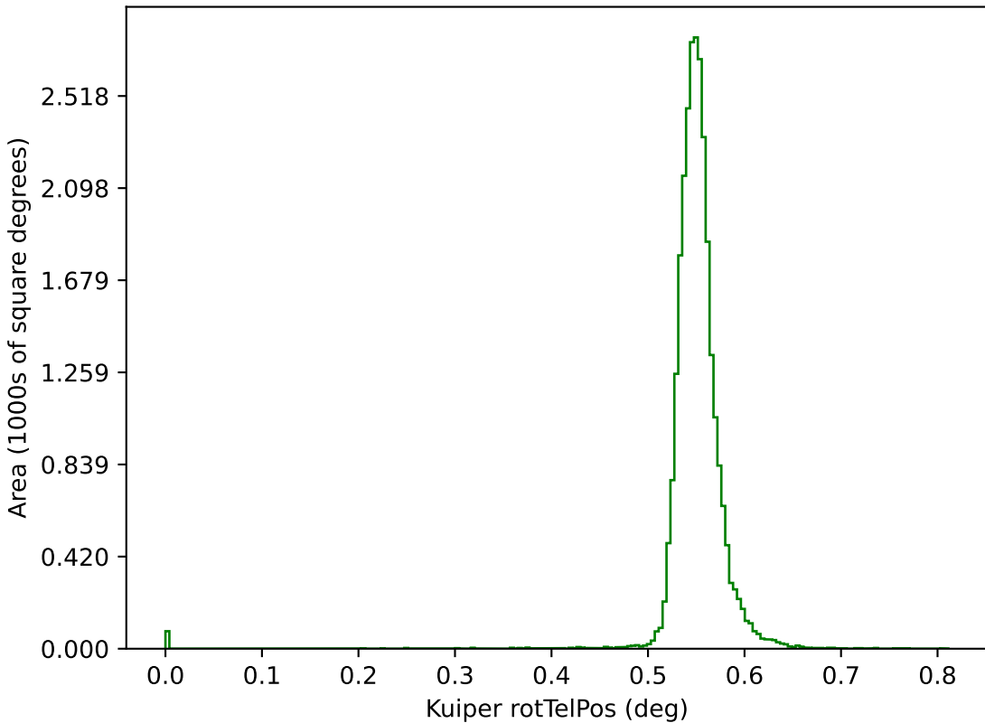
extra_ss_neo3_v3.4_10yrs g: Kuiper rotTelPos
