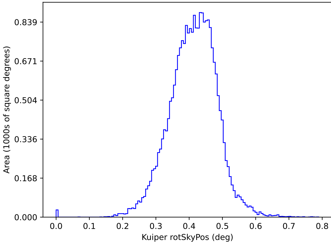
extra_ss_neo3_v3.4_10yrs y: Kuiper rotSkyPos
