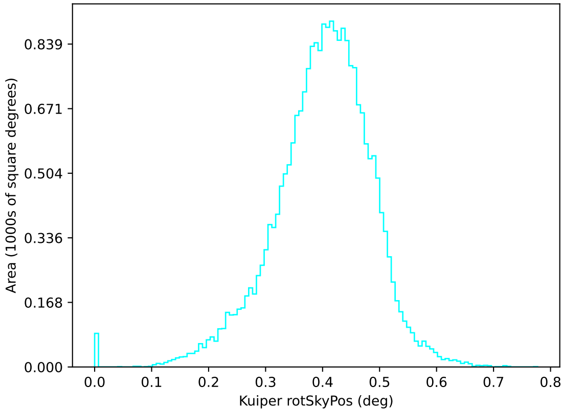
extra_ss_neo3_v3.4_10yrs u: Kuiper rotSkyPos
