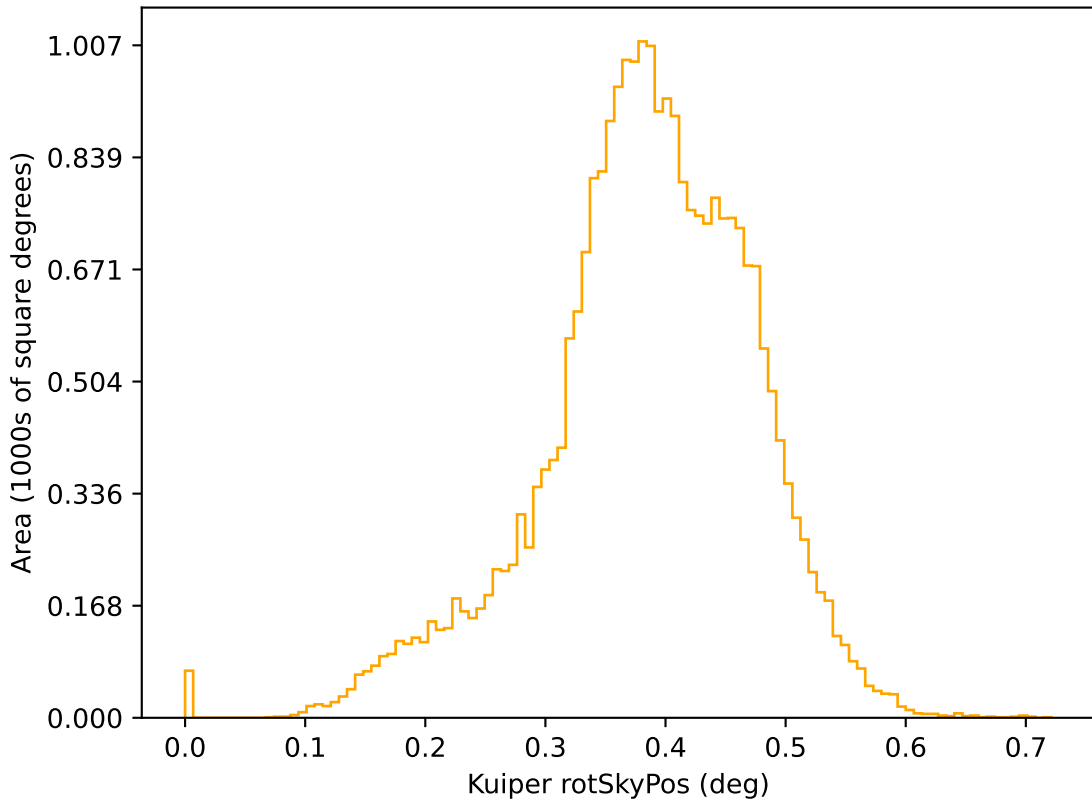
extra_ss_neo3_v3.4_10yrs r: Kuiper rotSkyPos
