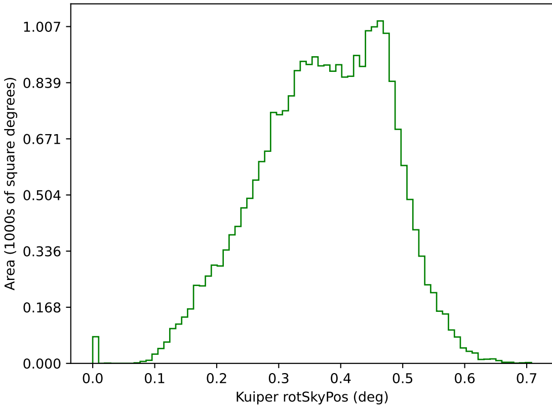
extra_ss_neo3_v3.4_10yrs g: Kuiper rotSkyPos
