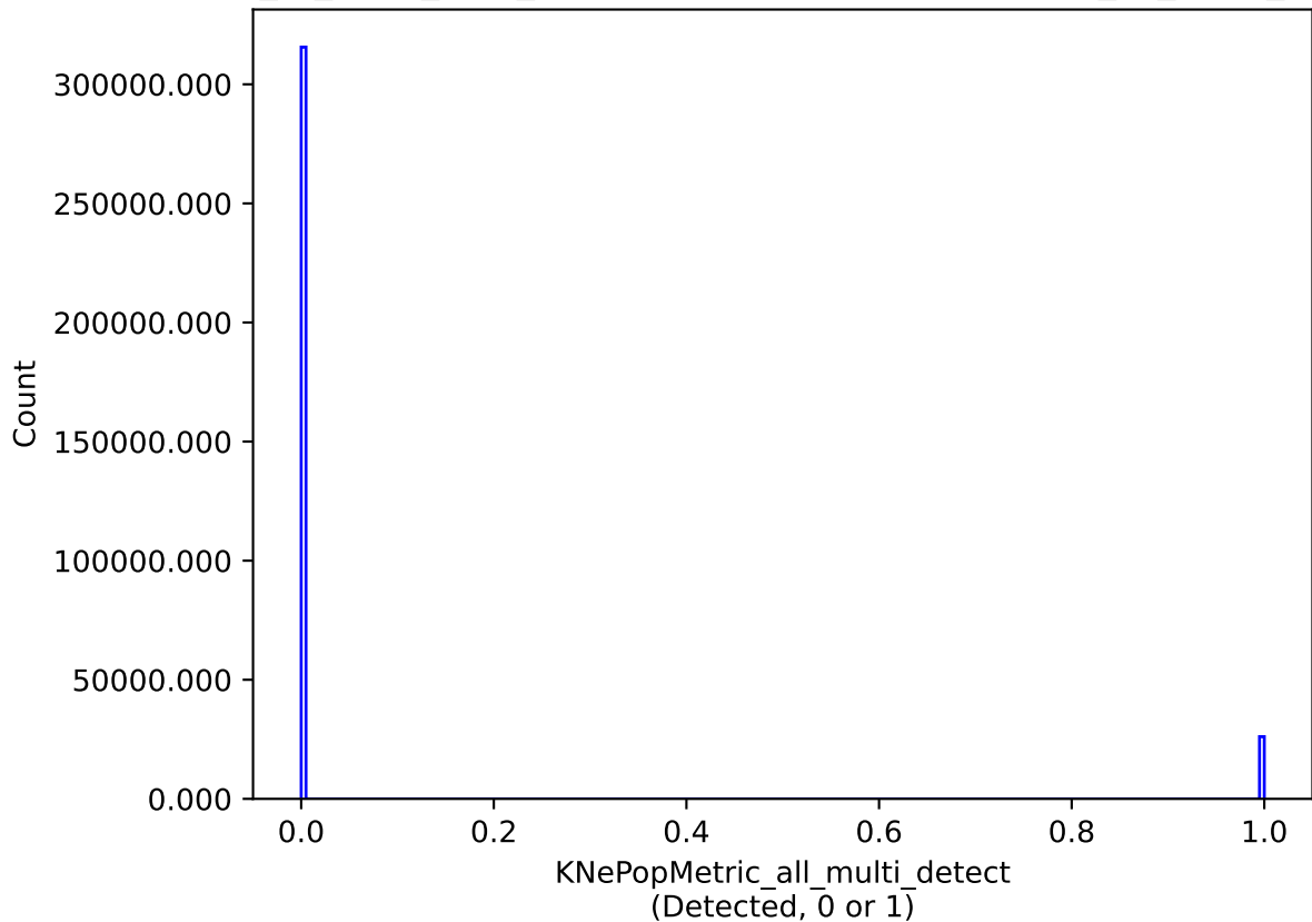
extra_ss_neo3_v3.4_10yrs all models: KNePopMetric_all_multi_detect
