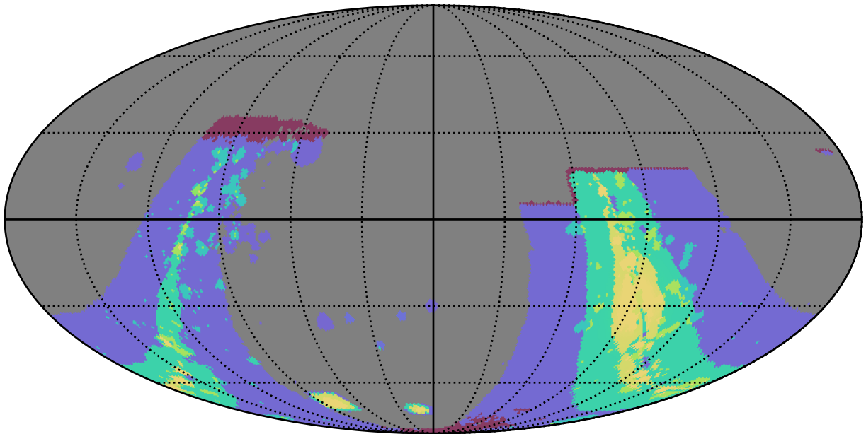
extra_ss_neo3_v3.4_10yrs : GalplaneFootprintMetric_combined_map_Tau_73_0
