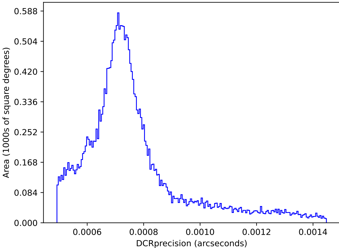
extra_ss_neo3_v3.4_10yrs : DCRprecision
