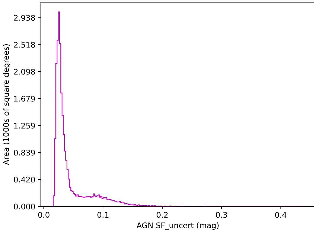
extra_ss_neo3_v3.4_10yrs z band: AGN SF_uncert
