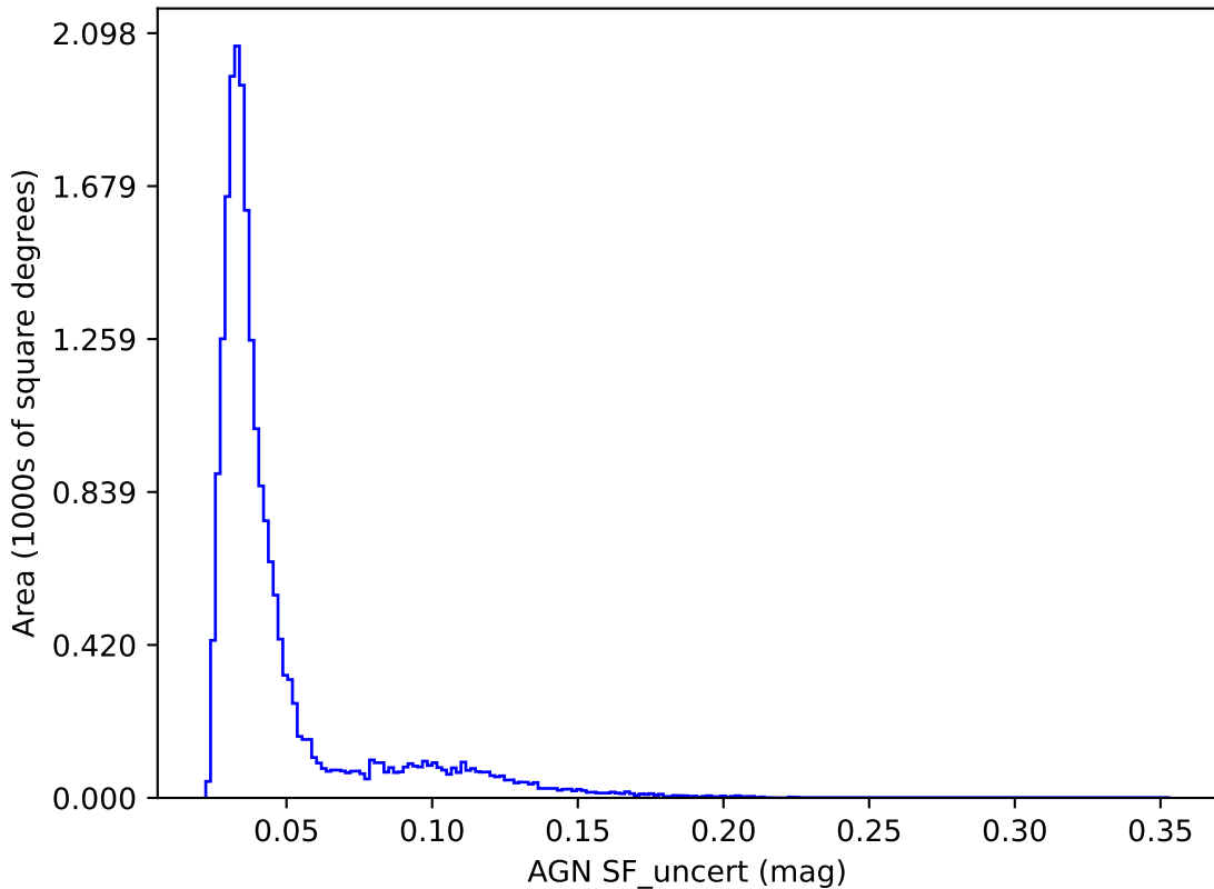
extra_ss_neo3_v3.4_10yrs y band: AGN SF_uncert
