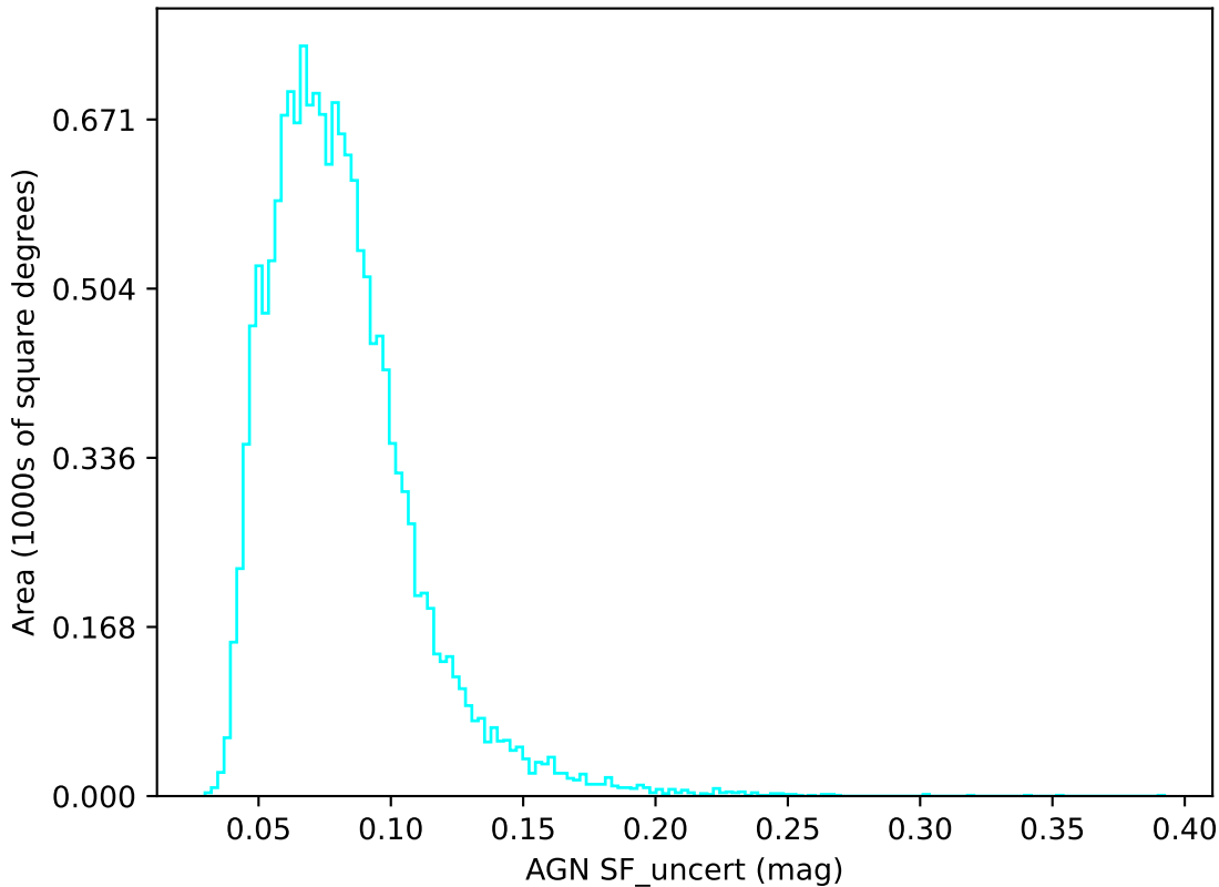
extra_ss_neo3_v3.4_10yrs u band: AGN SF_uncert
