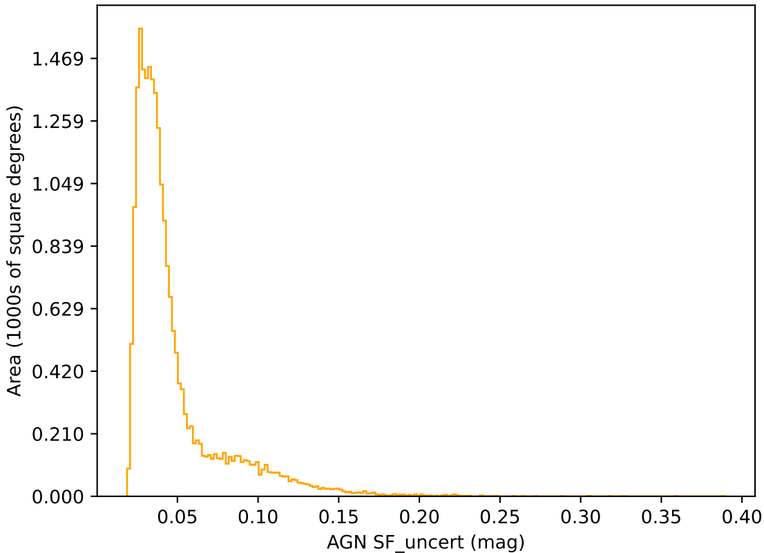
extra_ss_neo3_v3.4_10yrs r band: AGN SF_uncert
