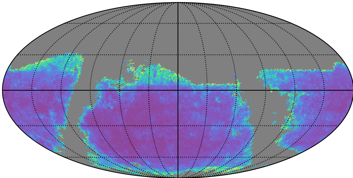
extra_ss_neo3_v3.4_10yrs g band: AGN SF_uncert
