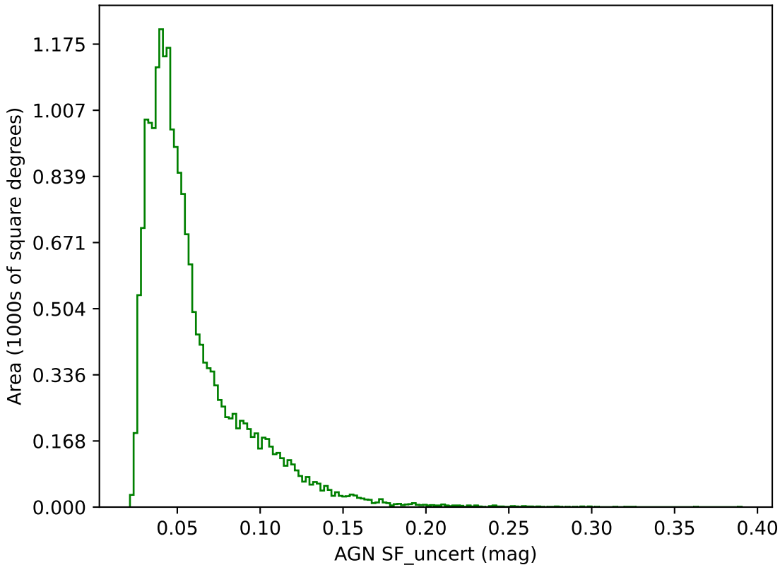
extra_ss_neo3_v3.4_10yrs g band: AGN SF_uncert
