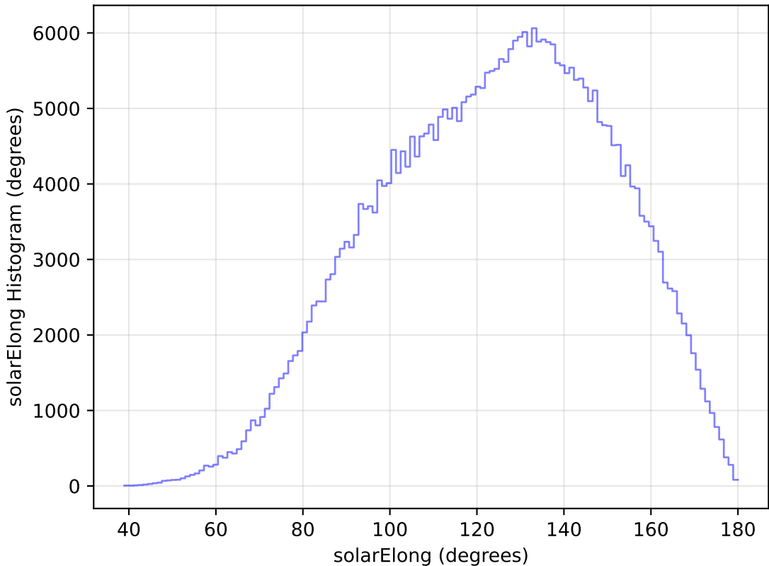
extra_ss_neo3_v3.4_10yrs WFD y band: solarElong Histogram
